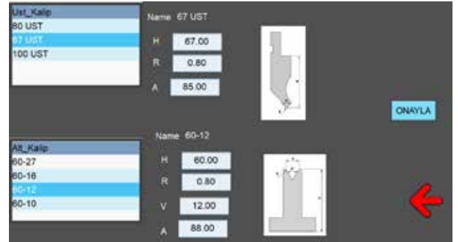
Kalip Seçim ve Oluşturma Özelliği Selection and Drawing Tooling Feature on Controller
