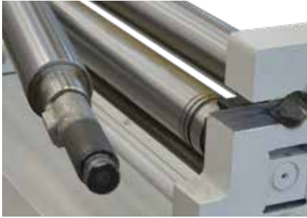
Standart Elle Açılabilir Sac Çıkarma Kafası Standard Manual Dropend
